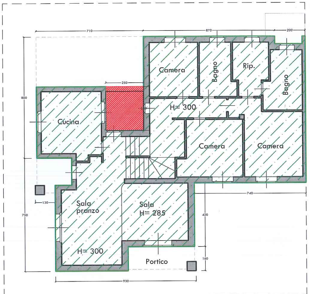
PIANO TERRA - RILIEVO
